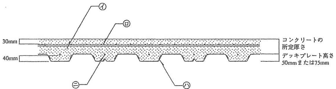
B-B断面図
