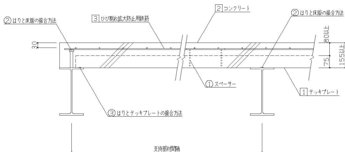
C-C 断面図
