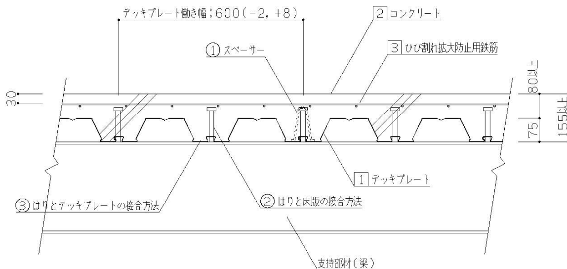
A-A 断面図
