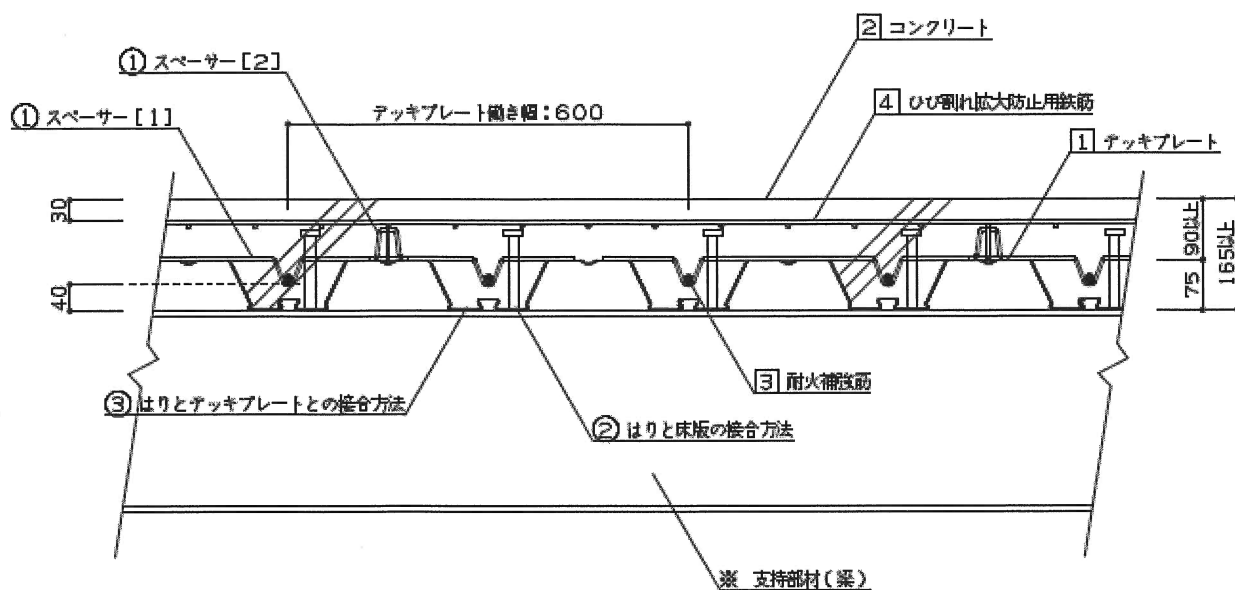
A-A 断面図
