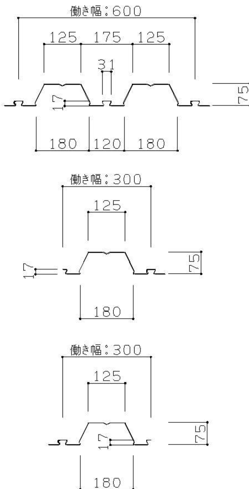
デッキプレート断面図
