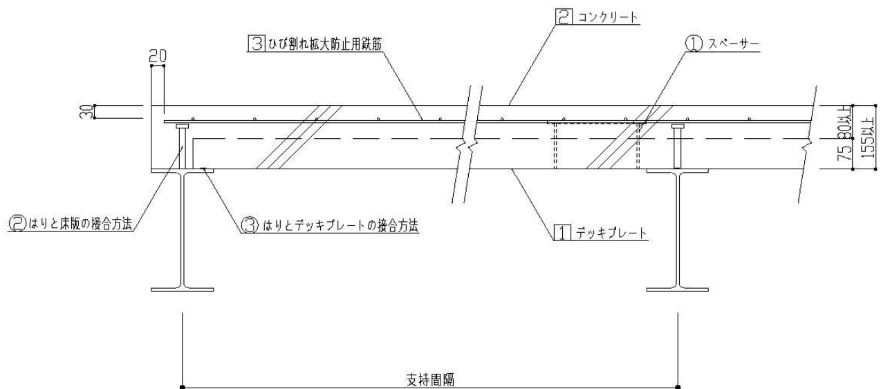
B－B 断面図（連続支持）
