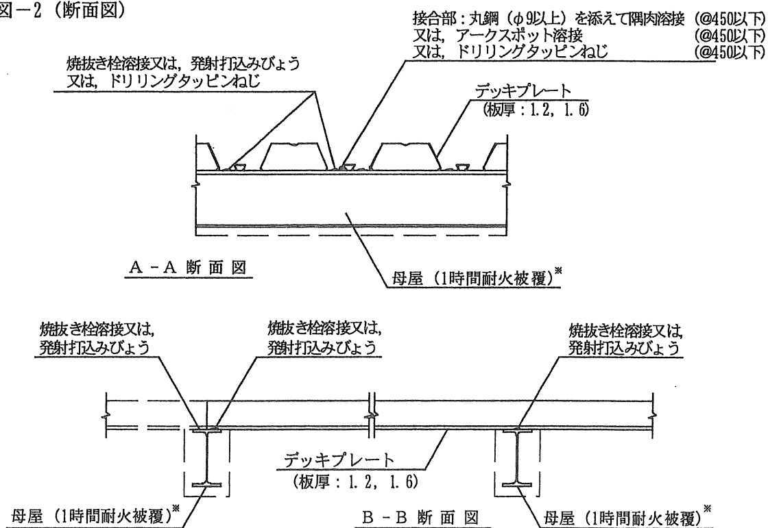
別図－2（断面図）
