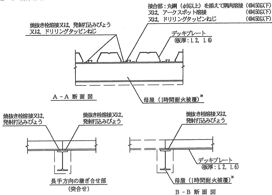
別図－2（断面図）
